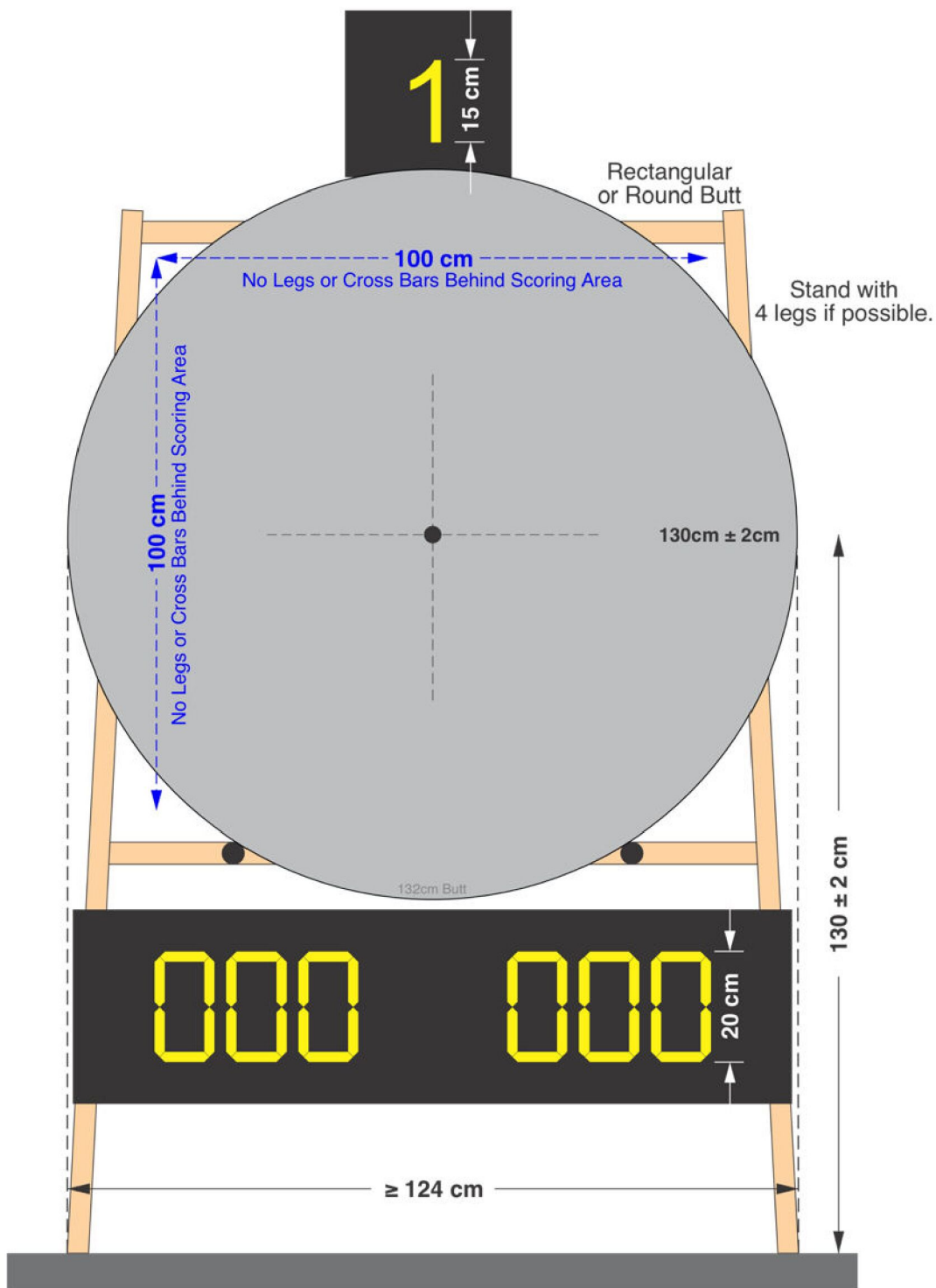
Obrázok 6: Nastavenie vnútornej terčovnice
